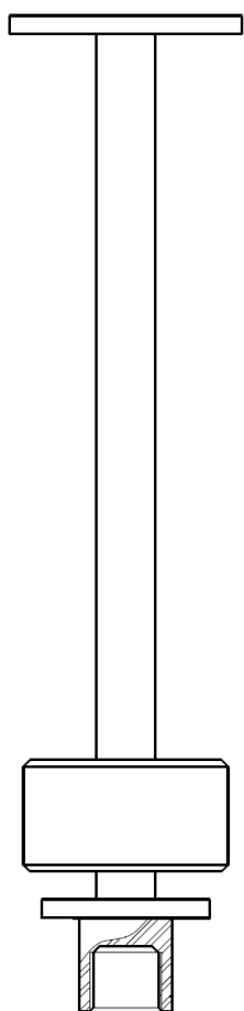
FIGURA 2 – Haste do êmbolo
