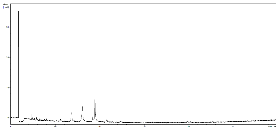
Figura 7- Cromatograma da condição cromatográfica 1: gradiente linear de 5-100% de ACN (B) em 60 min, vazão 1mL/min, \lambda=280 nm, V_{inj.} = 10\mu\text{L} .
