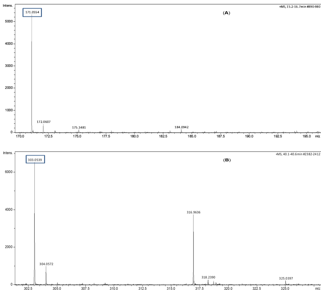
Figura 10: ESI(+)-MS ampliado do EACPG. [M+H]^+ em m/z 171 – ácido gálico (A) e [M+H]^+ em m/z 303 – ácido elágico.
