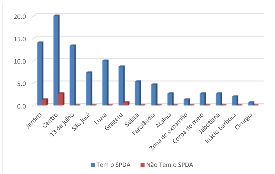
Figura 15 – Sistema de para-raios(SPDA) das edificações vistoriadas pelo CBMSE. 2013
