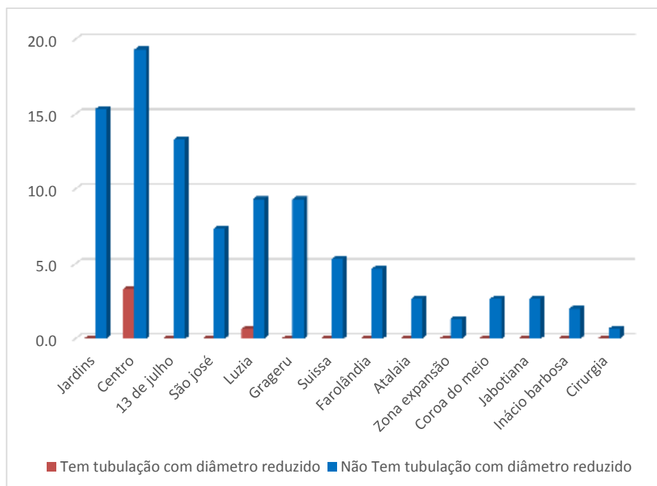
Figura 63 – Existência de tubulação do sistema contra incêndio com diâmetro reduzido
