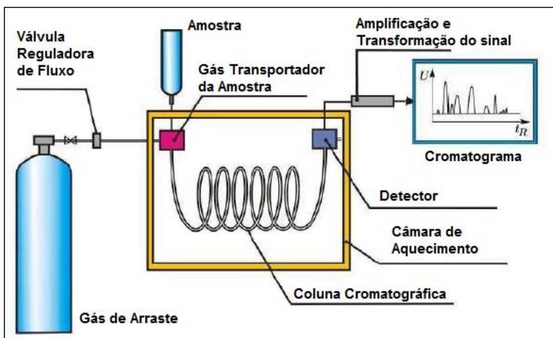
Figura 11 - Sistema simplificado de um Cromatógrafo a Gás.
