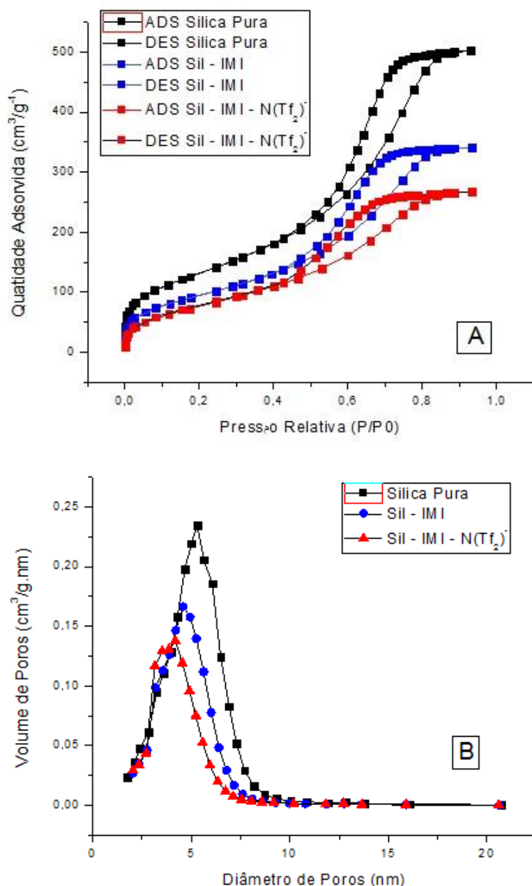
Figura 14 - (A) Isoterma de adsorção/dessorção N 2 e (B) distribuição do tamanho de poro da Sílica pura, Sil-IMI e Sil-IMI-N(Tf 2 ) - .
