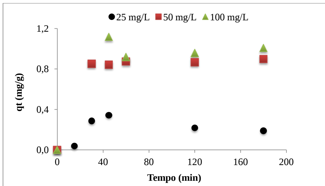
Figura 17- Capacidade de adsorção do dibenzotiofeno em Sil-IMI-N(Tf 2 ) - versus tempo de adsorção em diferentes concentrações iniciais. Condições: T= 40°C, m_{\text{adsorvente}} = 300 mg.
