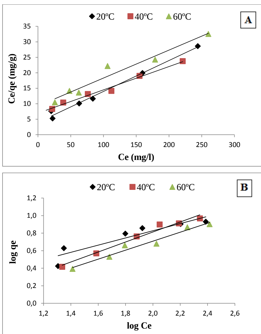
Figura 21 - Isotermas de adsorção de (A) Langmuir e de (B) Freundlich para o dibenzotiofeno sobre Sil-IMI-N(Tf 2 ) a diferentes temperaturas. Condições: tempo de equilíbrio= 24 h, m adsorvente = 300 mg.
