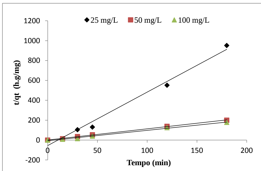
Figura 20 - Cinética pseudo-segunda ordem para adsorção do dibenzotiofeno Sil-IMI-N(Tf 2 ) - em função do tempo, a várias concentrações iniciais. Condições: T= 40°C, m adsorvente = 300 mg.
