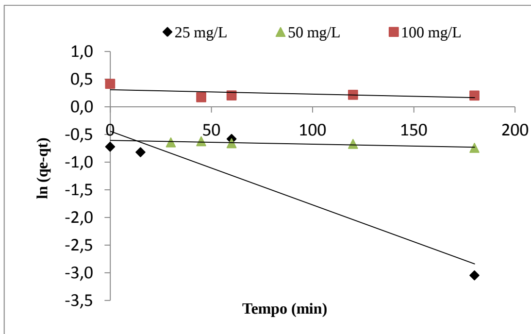
Figura 19 - Cinética pseudo-primeira ordem para adsorção do dibenzotiofeno Sil-IMI-N(Tf2) - em função do tempo, a várias concentrações iniciais. Condições: T= 40°C, m_{\text{adsorvente}} = 300 mg.
