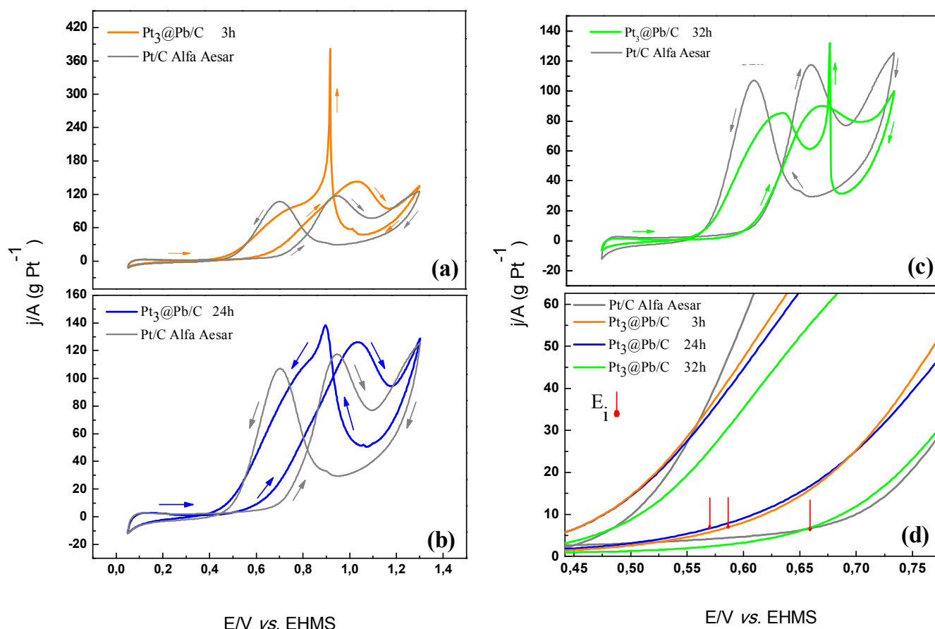
Figura 4. Voltamogramas cíclicos obtidos (segundo ciclo) em solução aquosa de 0,5 mol L -1 de H 2 SO 4 + 0,5 mol L -1 de etanol a 20 mV s -1 , para os eletrocatalisadores Pt 3 @Pb/C MRS preparados sob diferentes tempos de agitação: (a) 3 h (—); (b) 24 h (—); e (c) 32 h (—) e Pt/C Alfa Aesar (—). (d) Comparação dos valores de E_i para todos eletrocatalisadores. As setas indicam a direção de varredura de potencial.
