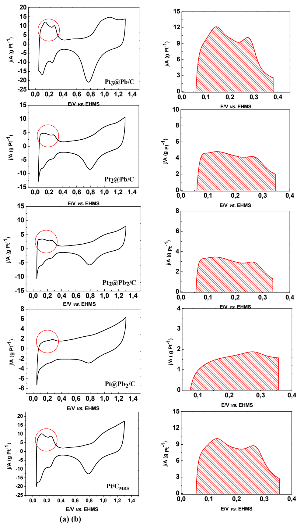
Figura 24. (a) Voltamogramas cíclicos dos catalisadores \text{Pt}_3@\text{Pb} , \text{Pt}_2@\text{Pb}_2 , \text{Pt}_2@\text{Pb} e \text{Pt}@\text{Pb}_2 e \text{Pt}/\text{C}_{\text{MRS}} em solução de \text{H}_2\text{SO}_4 0,5 mol \text{L}^{-1} , a temperatura de 25 °C e \nu = 20 \text{ mV s}^{-1} com a região pela qual foi calculada a carga de oxidação do hidrogênio assinalada. (b) Ampliação da área pela qual foi calculada a carga de oxidação do hidrogênio.
