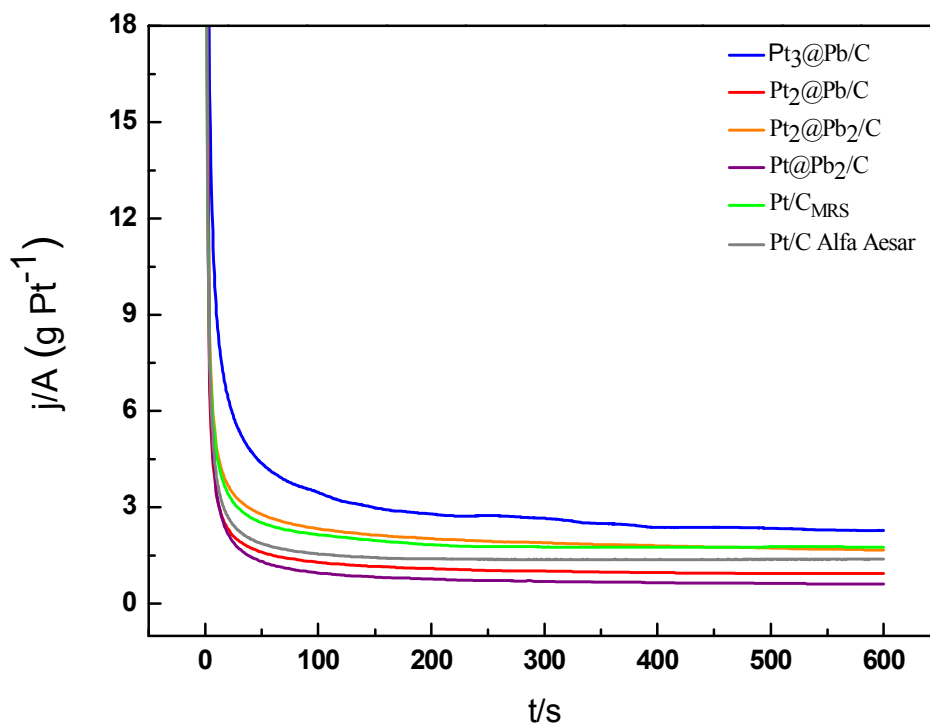
Figura 86. Cronoamperogramas obtidos para os eletrocatalisadores \text{Pt}_3@\text{Pb}/\text{C} , \text{Pt}_2@\text{Pb}/\text{C} , \text{Pt}_2@\text{Pb}_2/\text{C} , \text{Pt}@\text{Pb}_2/\text{C} , \text{Pt}/\text{C}_{\text{MRS}} e \text{Pt}/\text{C} Alfa Aesar em solução aquosa de 0,5 \text{ mol L}^{-1} \text{ H}_2\text{SO}_4 + 0,5 \text{ mol L}^{-1} de etanol. Eletrodos polarizados a 0,5 \text{ V} .
