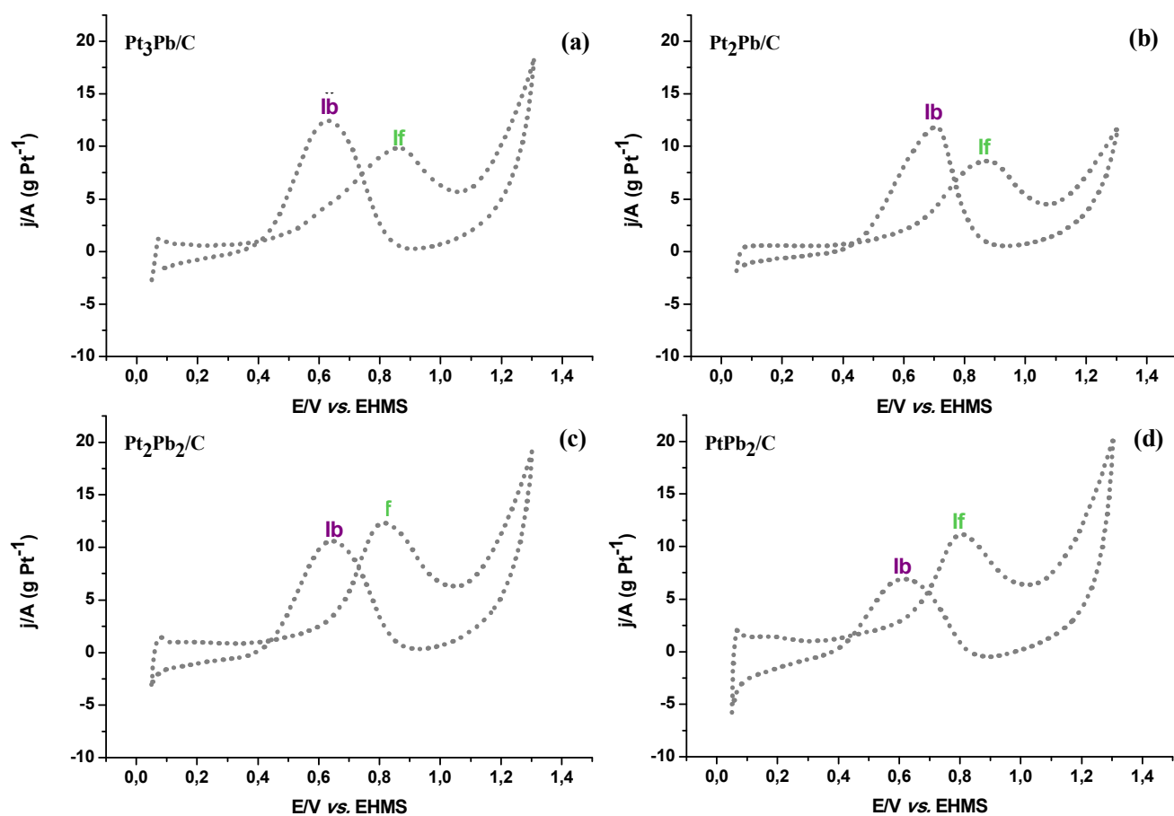
Figura 31. Voltamogramas cíclicos para a oxidação de glicerol sobre eletrocatalisadores de liga baseados em Pt e Pb: (a) \text{Pt}_3\text{Pb} , (b) \text{Pt}_2\text{Pb} , (c) \text{Pt}_2\text{Pb}_2 , (d) \text{PtPb}_2 em solução de \text{H}_2\text{SO}_4 0,5 \text{ mol L}^{-1} + 0,5 \text{ mol L}^{-1} de glicerol. \nu = 20 \text{ mV s}^{-1} .
