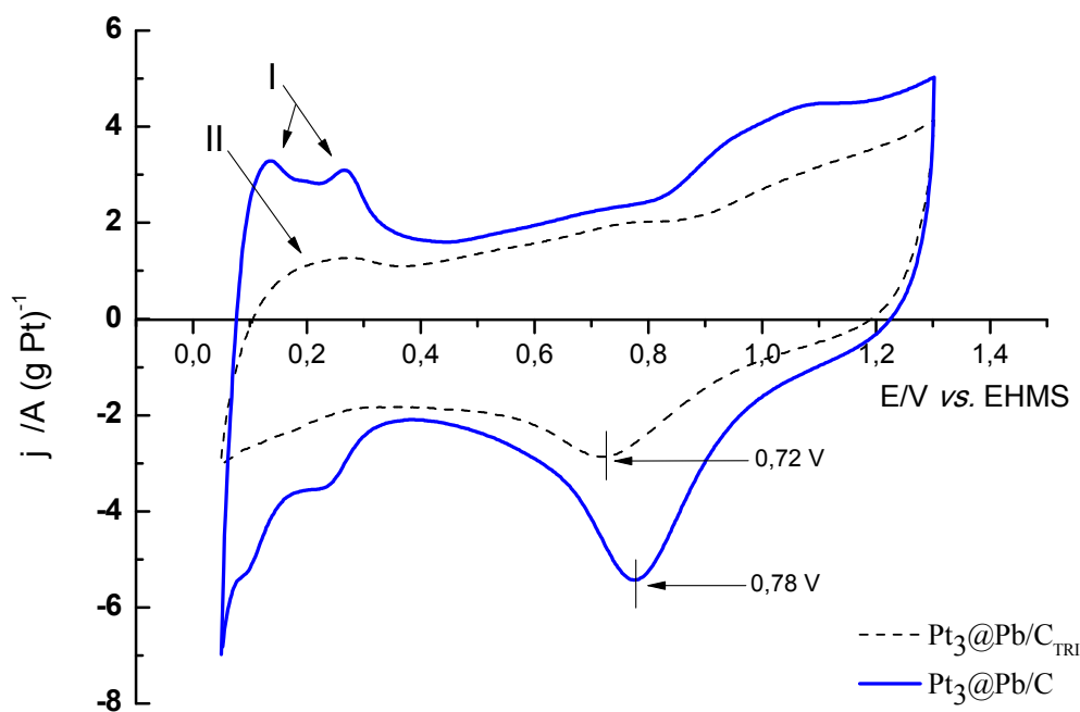
Figura 14. Voltamogramas cíclicos (segundo ciclo) para os electrocatalisadores \text{Pt}_3@\text{Pb}/\text{C}_{\text{TRI}} (---) e \text{Pt}_3@\text{Pb}/\text{C} (—) preparados por MRS obtidos a uma velocidade de 20 \text{ mV s}^{-1} em solução de 0,5 \text{ mol L}^{-1} \text{ H}_2\text{SO}_4 à temperatura de 25^\circ \text{C} .
