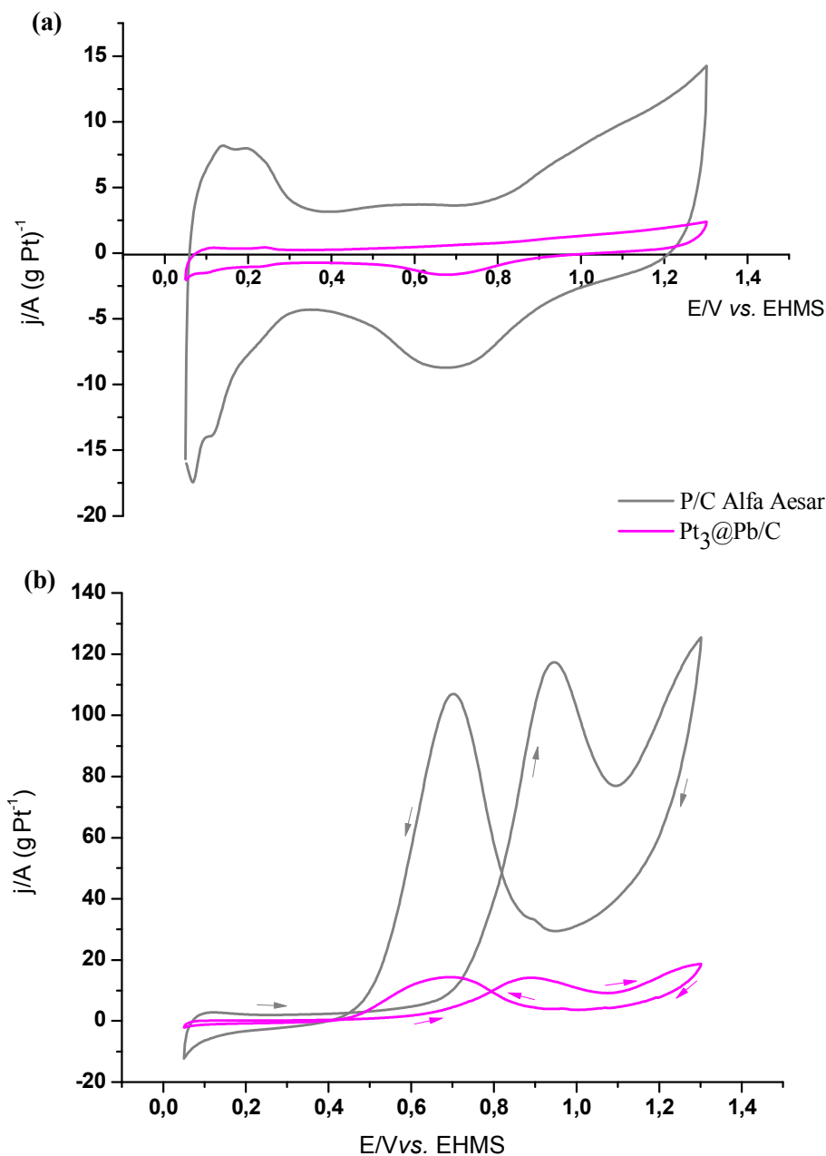
Figura 11. (a) Voltamogramas cíclicos obtidos (segundo ciclo) em solução aquosa de 0,5 \text{ mol L}^{-1} \text{H}_2\text{SO}_4 a 20 \text{ mV s}^{-1} e T = 25^\circ\text{C} para os eletrocatalisadores Pt/C Alfa Aesar (—) e \text{Pt}_3@\text{Pb}/\text{C} (—) preparado via redução por borohidreto. (b) Voltamogramas obtidos na presença de 0,5 \text{ mol L}^{-1} de etanol. As setas indicam a direção de varredura de potencial.
