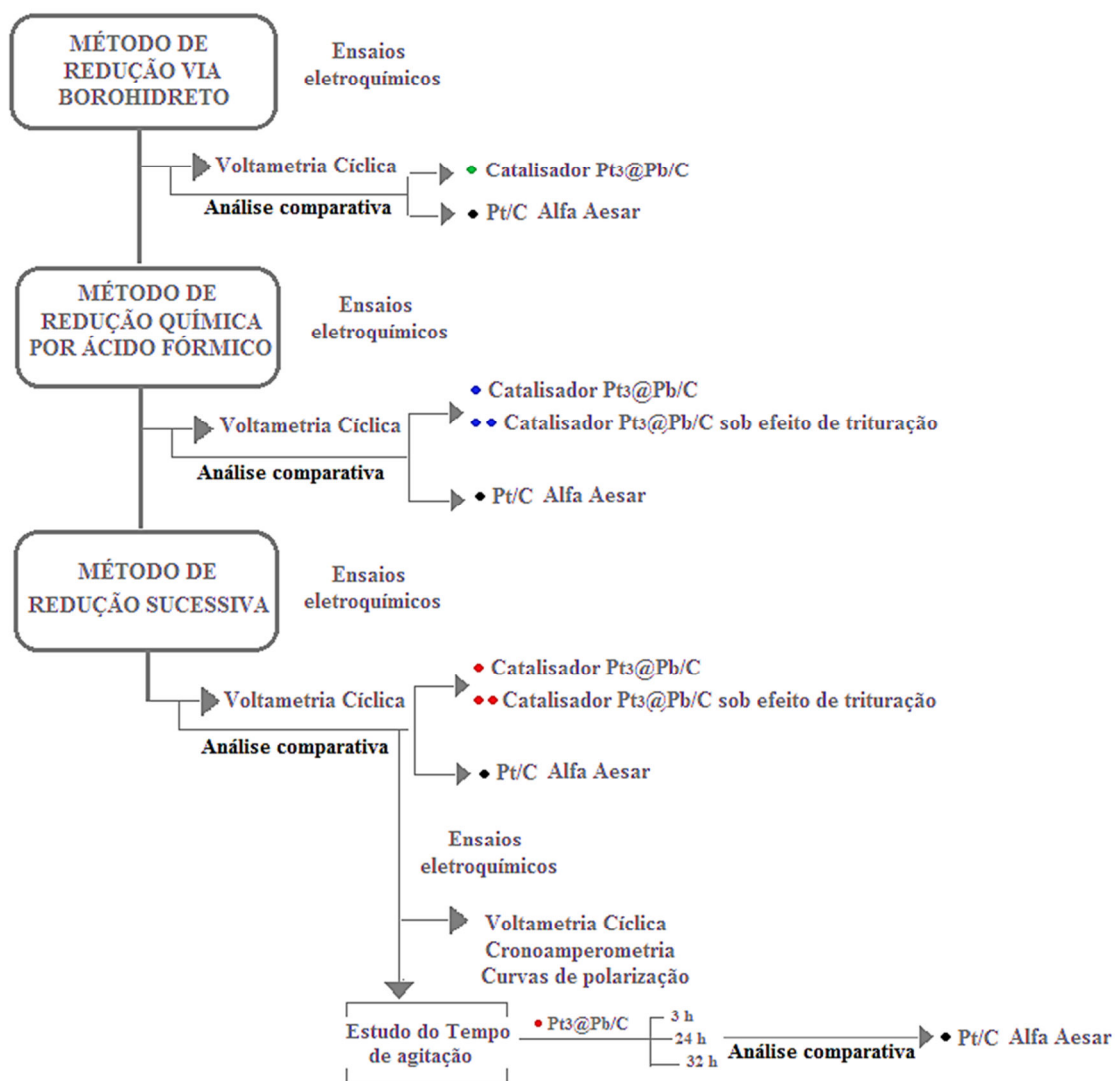
Figura 4. Fluxograma dos métodos utilizados na preparação do eletrocatalisador \text{Pt}_3\text{@Pb/C} para aplicação na oxidação de etanol.
