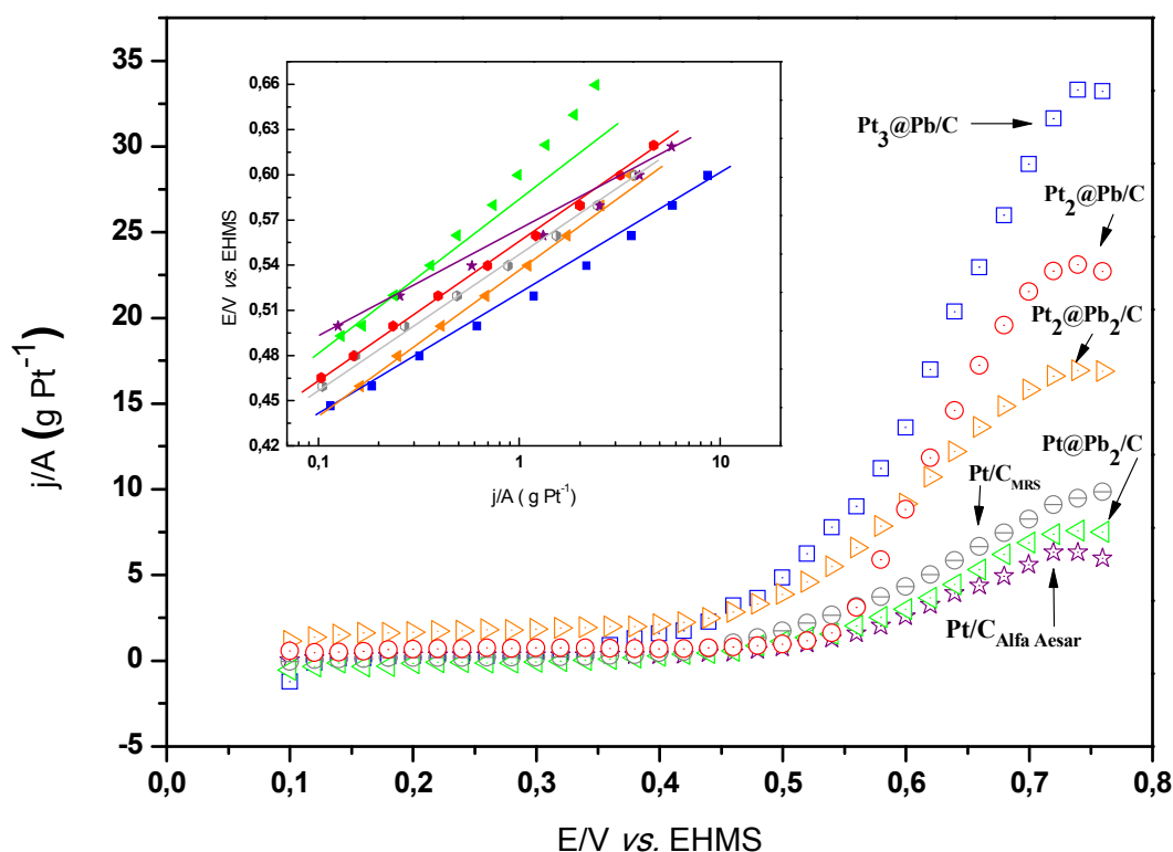
Figura 98. Curvas de polarização em estado quase-estacionário obtidos a partir de curvas de polarização dos electrocatalisadores casca-núcleo: \text{Pt}_3@\text{Pb}/\text{C} , \text{Pt}_2@\text{Pb}/\text{C} , \text{Pt}_2@\text{Pb}_2/\text{C} , \text{Pt}@\text{Pb}_2/\text{C} , de \text{Pt}/\text{C}_{\text{MRS}} e \text{Pt}/\text{C} Alfa Aesar, com valores de corrente potencioestática medida após 200 s a cada 20 mV, em solução 0,5 mol L -1 de H 2 SO 4 e de etanol 0,5 mol L -1 . Inserção: Diagramas de Tafel correspondentes a cada uma das curvas de polarização.
