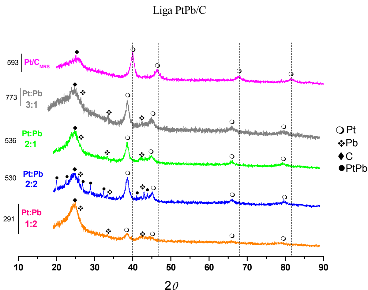
Figura 22. Difratomogramas de raios X para os catalisadores liga: \text{Pt}_3\text{Pb/C} , \text{Pt}_2\text{Pb/C} , \text{Pt}_2\text{Pb}_2/\text{C} , \text{PtPb}_2/\text{C} e \text{Pt/C} , preparados por MRS.
