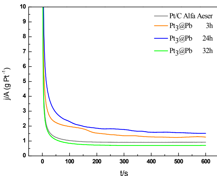
Figura 58. Cronoamperogramas obtidos para os eletrocatalisadores Pt 3 @Pb/C MRS preparados em tempos finais de agitação de 3 h (—), 24 h (—) e 32 h(—) e Pt/C Alfa Aesar (—) em solução aquosa de 0,5 mol L -1 de H 2 SO 4 + 0,5 mol L -1 de etanol. Eletrodos polarizados a 0,5 V.
