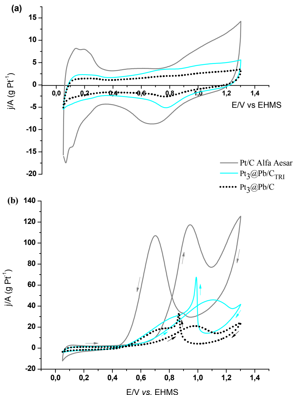
Figura 13. (a) Voltamogramas cíclicos obtidos (segundo ciclo) em solução aquosa de 0,5 mol L -1 H 2 SO 4 a 20 mV s -1 e T = 25 °C para os eletrocatalisadores Pt 3 @Pb/C TRI (—) e Pt 3 @Pb/C (···) preparados via redução por ácido fórmico (HCOOH) e Pt/C Alfa Aesar (—). (b) Voltamogramas obtidos na presença de 0,5 mol L -1 de etanol. As setas indicam a direção de varredura de potencial.
