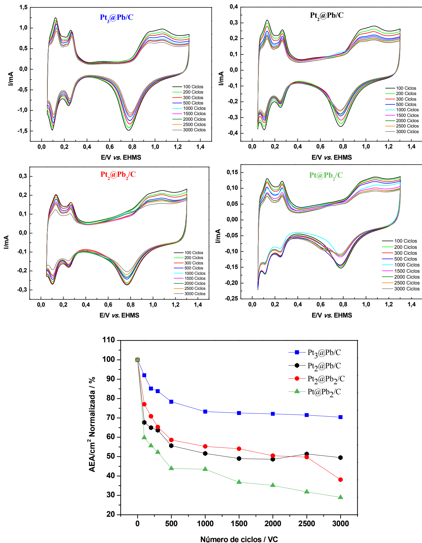
Figura 32. Estabilidade eletroquímica por VC para os catalisadores Pt 3 @Pb/C, Pt 2 @Pb/C, Pt 2 @Pb 2 /C e Pt@Pb 2 /C, com tempo total de ciclagem de 15 horas, em solução de 0,5 mol L -1 , \nu = 100 \text{ mV s}^{-1} .
